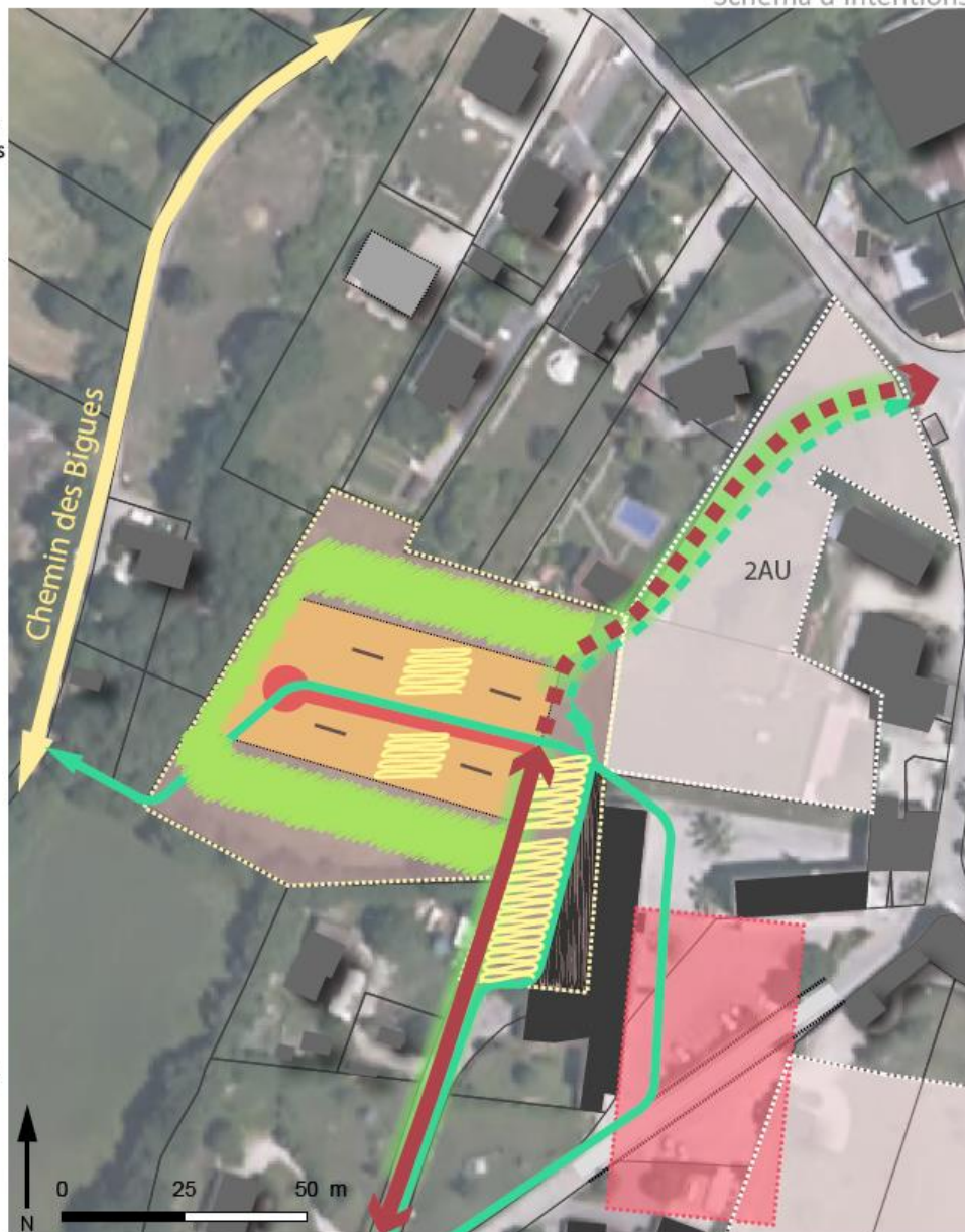
Schéma d'intentions
